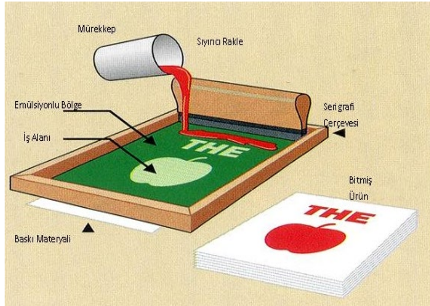
Görsel 2.27. Serigrafi Baskı Tekniği Çalışma Sistemi
