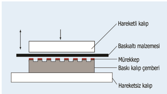
Görsel 2.29. Tipo Baskı Tekniği Çalışma Sistemi
