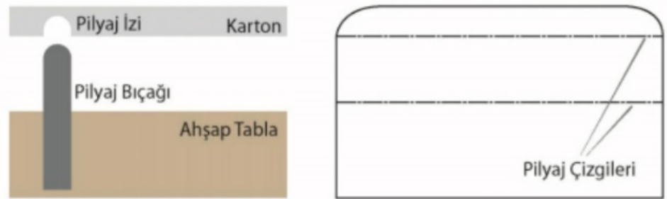
Görsel 2.21. Pilyaj uygulama tekniği
