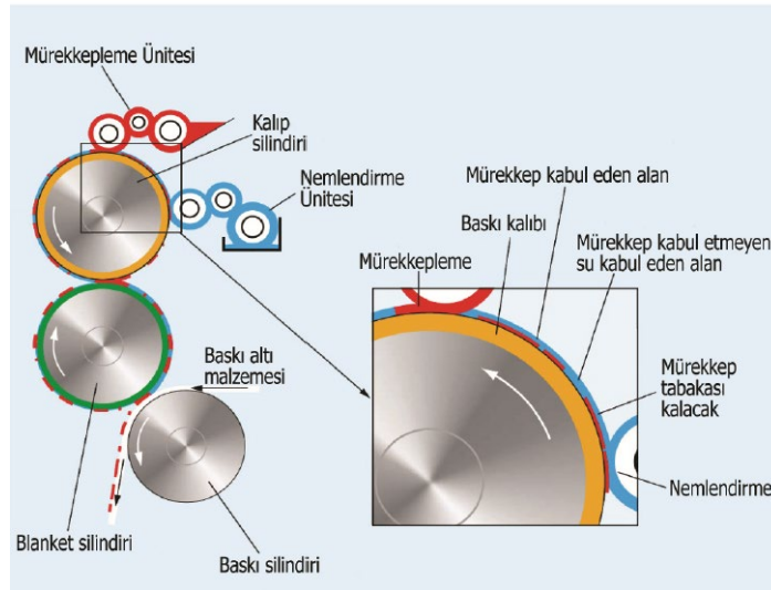
Görsel 2.17. Ofset Baskı Tekniği Çalışma Sistemi
